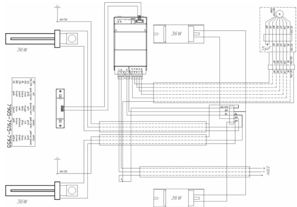
FIG. 6 externes Gebläse draußen (D 445999)
