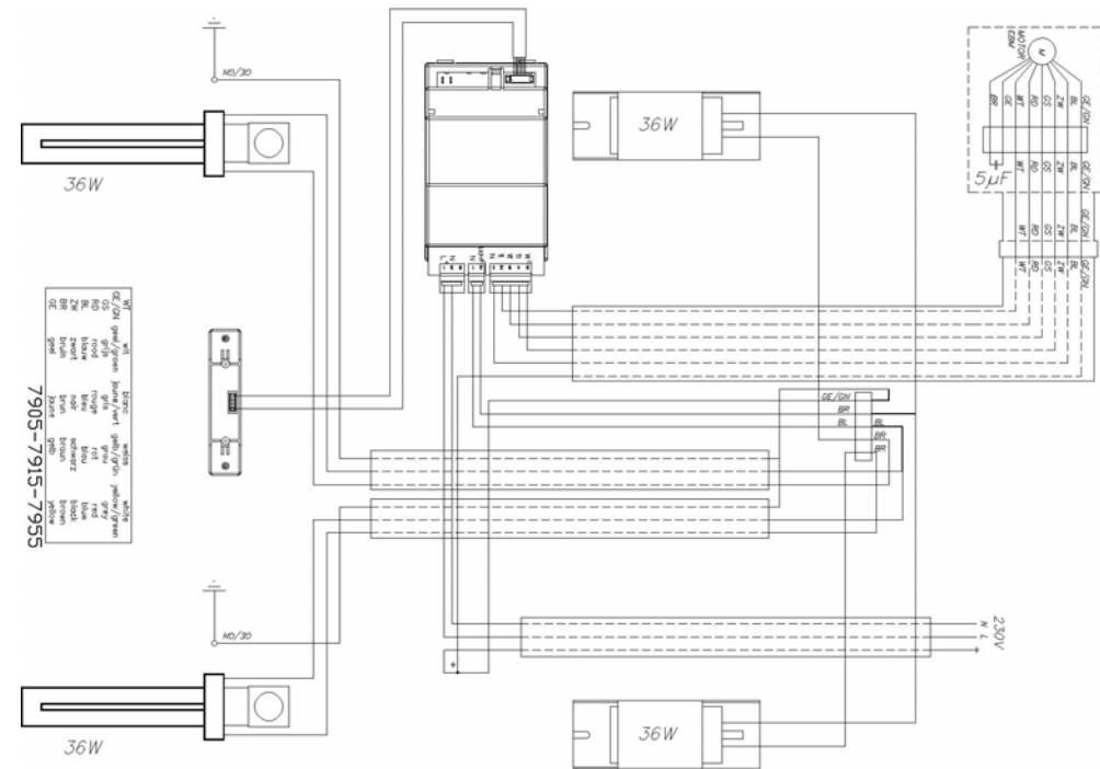
fig. 6 Motor op afstand buiten (D 445999)
