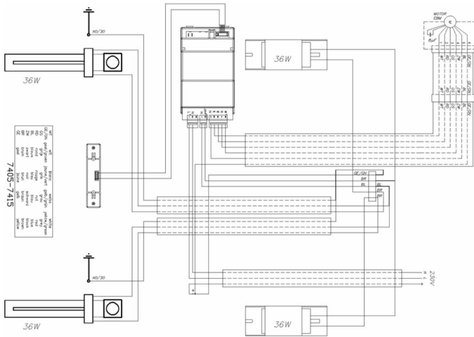
fig. 5 Motor op afstand binnen (D 345999)
